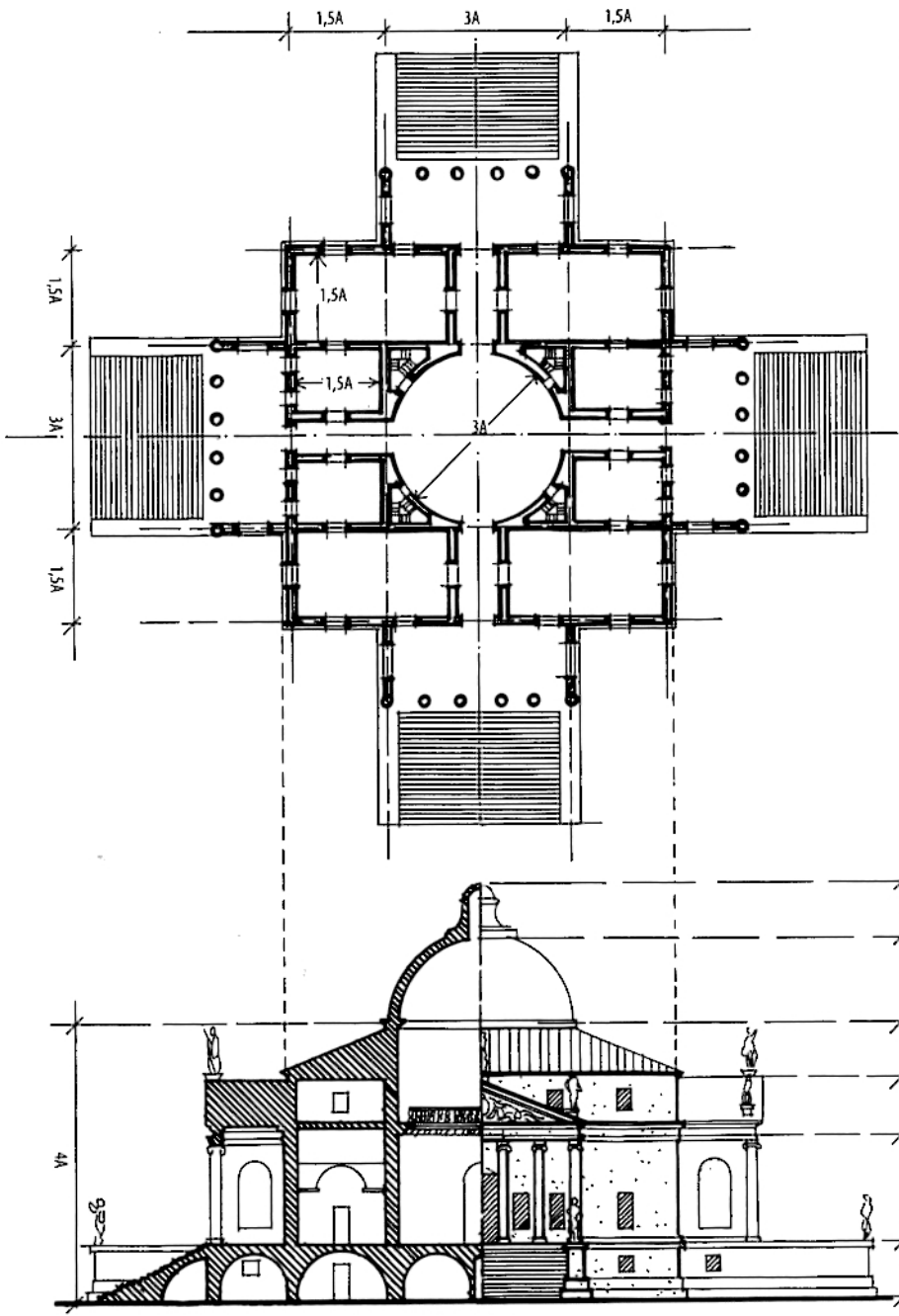
FIG. B-8 : Andrea Palladio, villa « Rotonda », Vicence (1565).
